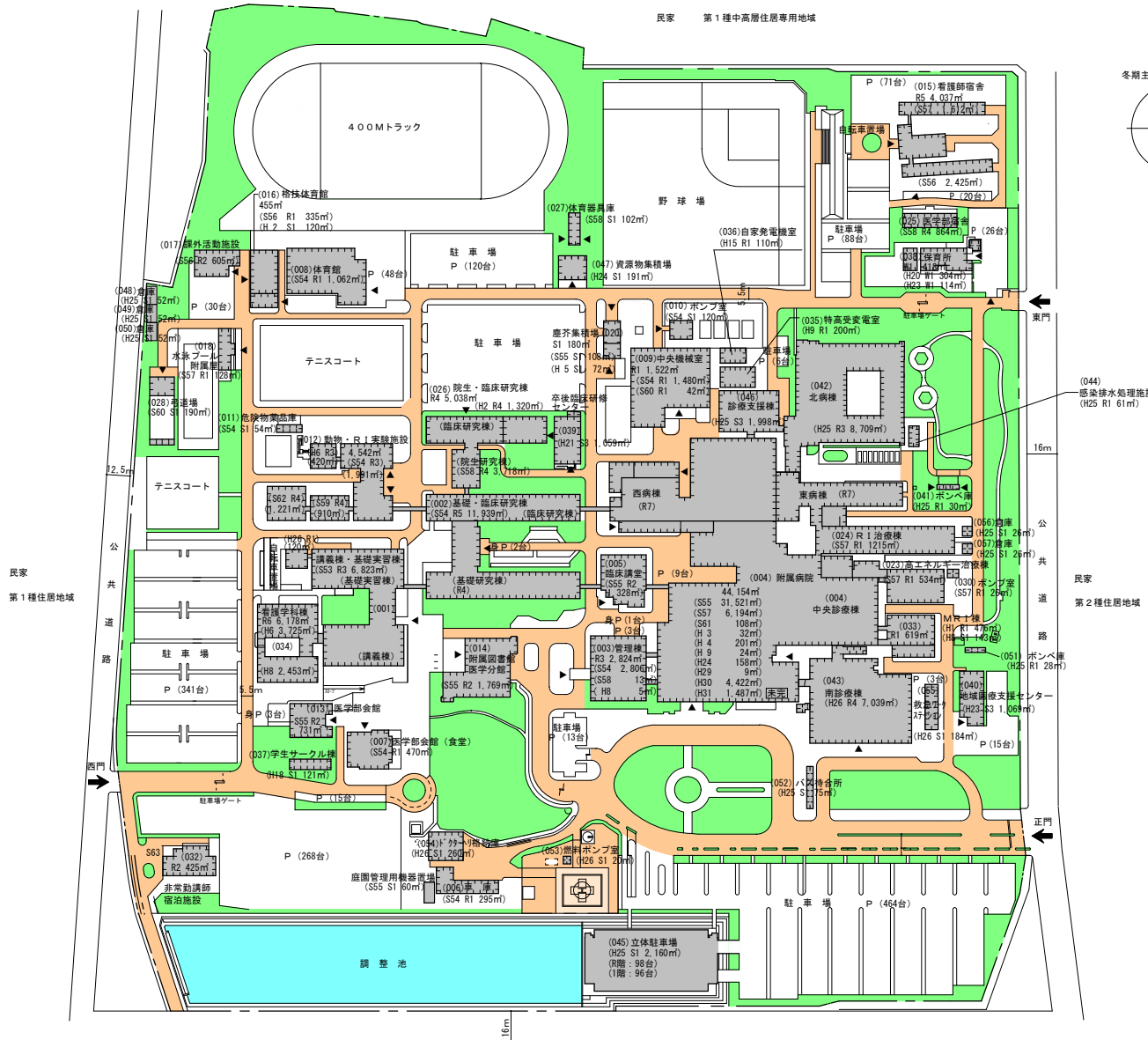
配置図 S=1/2,500
